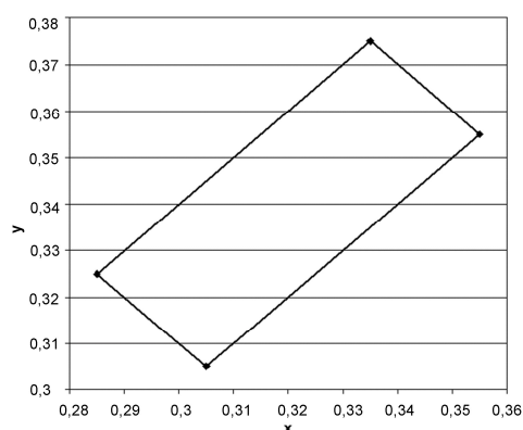
Rys. 1. Współrzędne chromatyczności x,y dla barwy żółtej oznakowania
